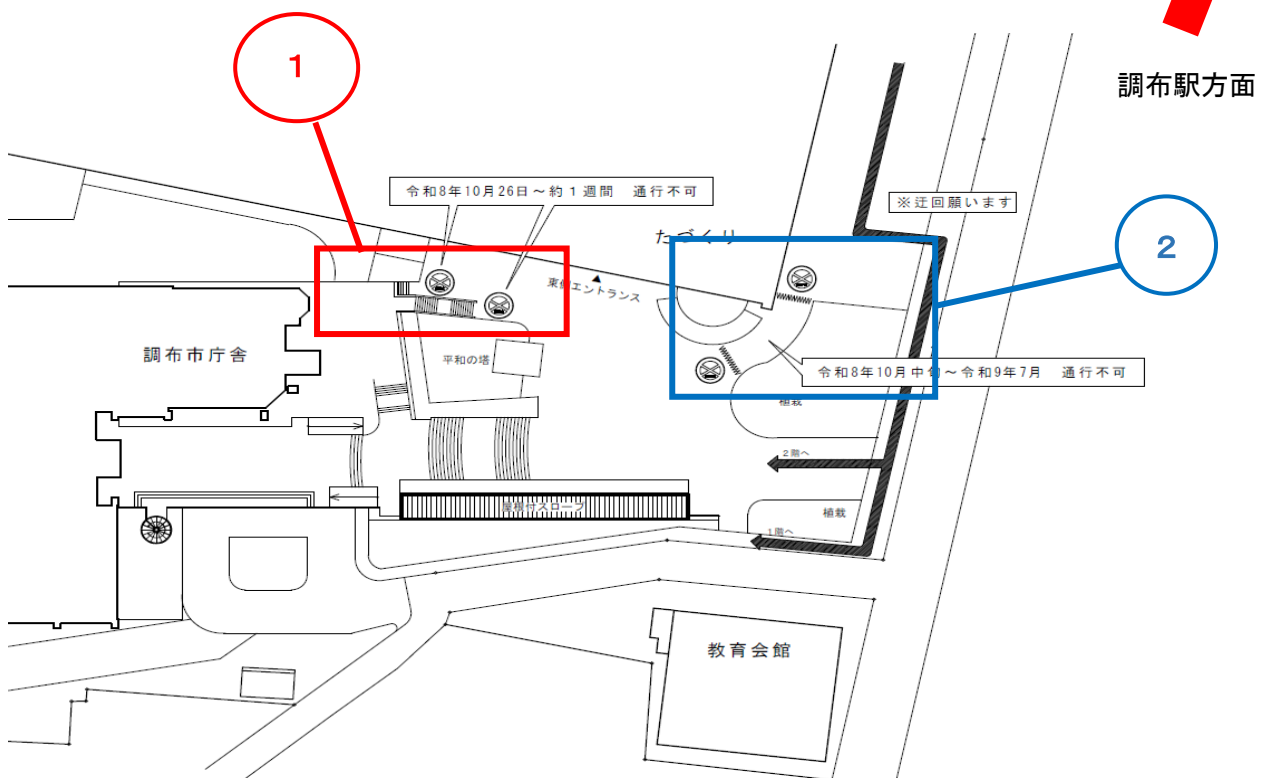
制限箇所予定図
